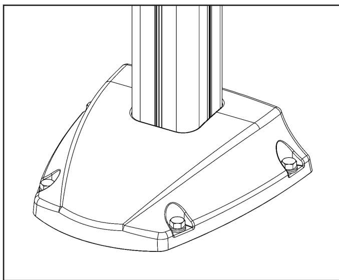
A,B,C y D Tornillos, arandelas y tacos estándar
